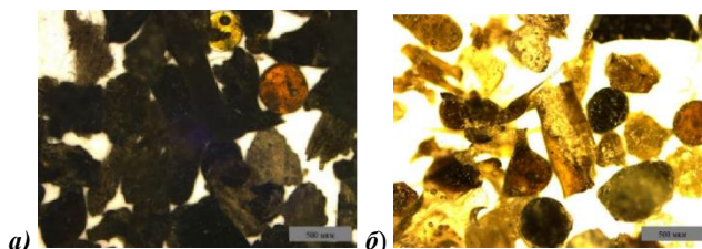
Рис. 1 Форма частиц отходов производства минеральной ваты ООО «Комбинат теплоизоляционных изделий» (г. Саранск) фракций: а – 0,63...1,25; б – 0,315...0,63
